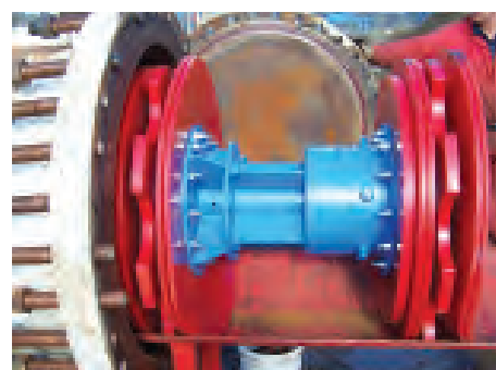
Одномодульный дисковый внутритрубный снаряд
