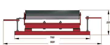
1R1C/800
